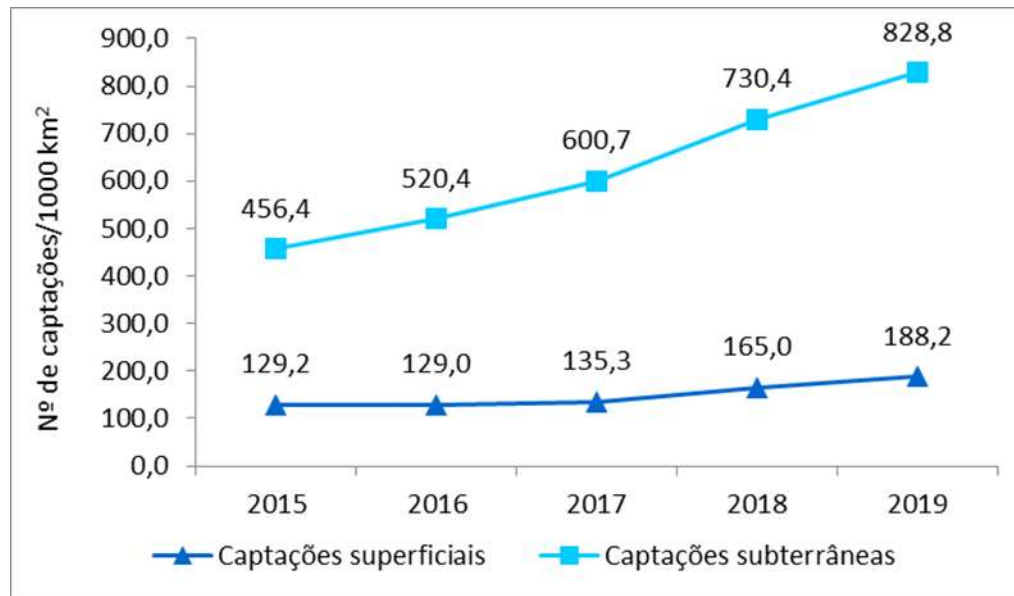
APÊNDICE 3.5.G Evolução de outorgas de captação superficial e subterrânea na UGRHI 06 (Fonte: DAEE, 2020 apud CBH-AT, 2020).
