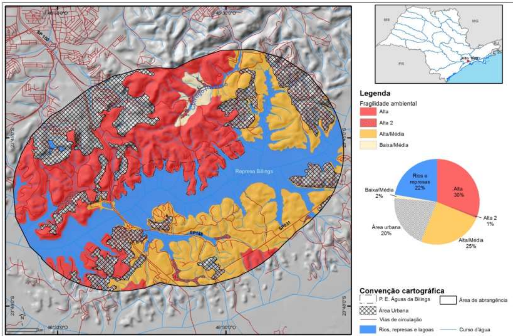
APÊNDICE 3.7.A Mapa de fragilidade potencial dos solos para a área de entorno do Parque Estadual Águas da Billings.
