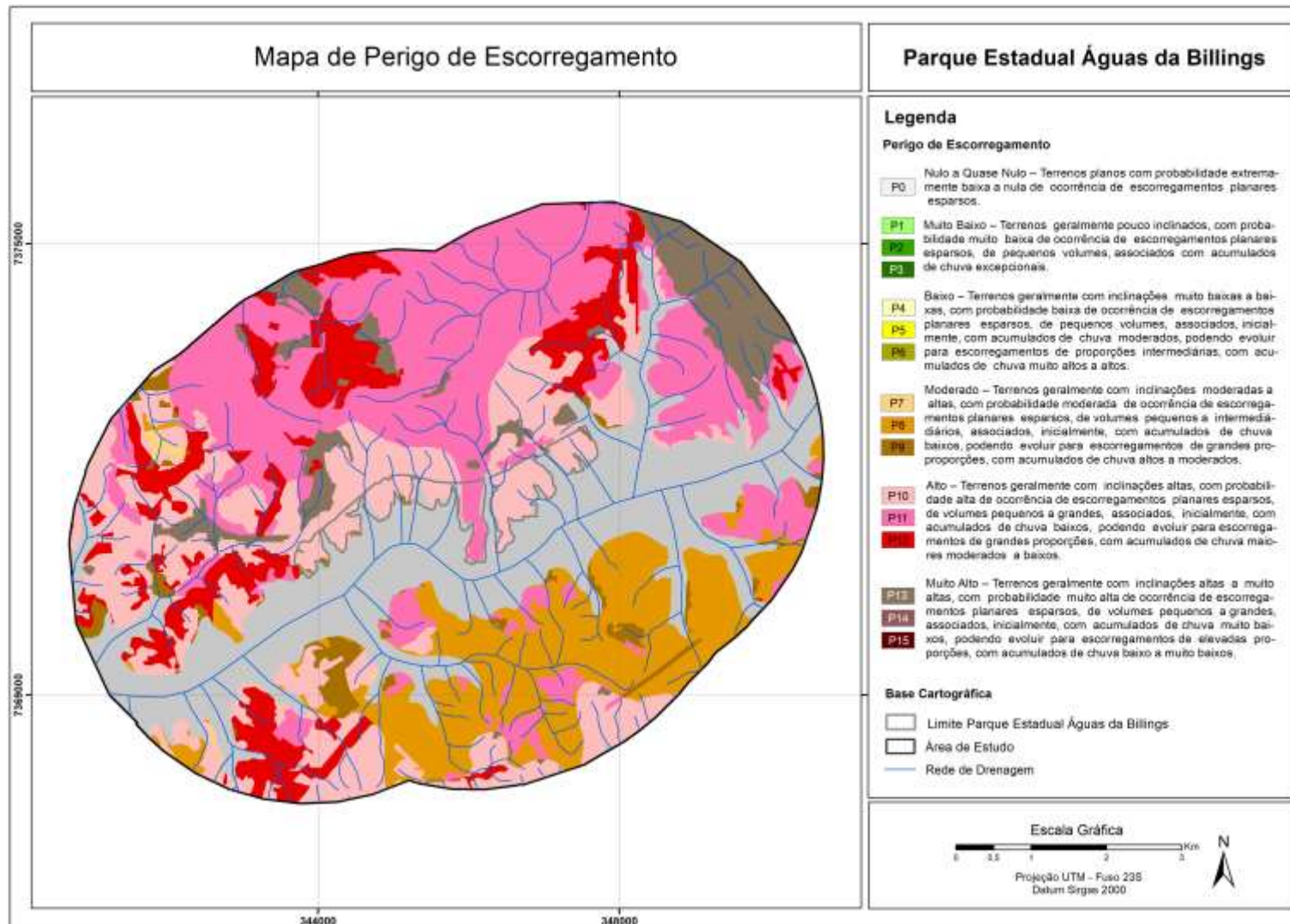
APÊNDICE 3.8.D Mapa de Perigo de Escorregamento Planar da área de estudo. Fonte: autores.
