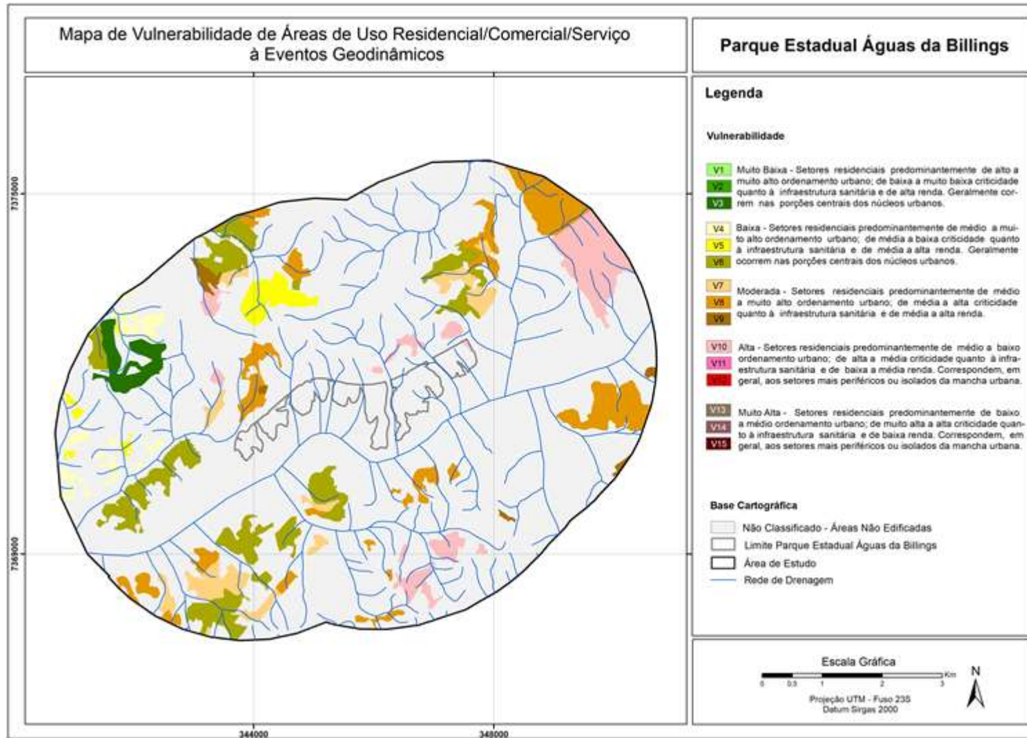
APÊNDICE 3.8.F Mapa de Vulnerabilidade de áreas uso do tipo Residencial/Comercial/Serviços da área de estudo. Fonte: autores.
